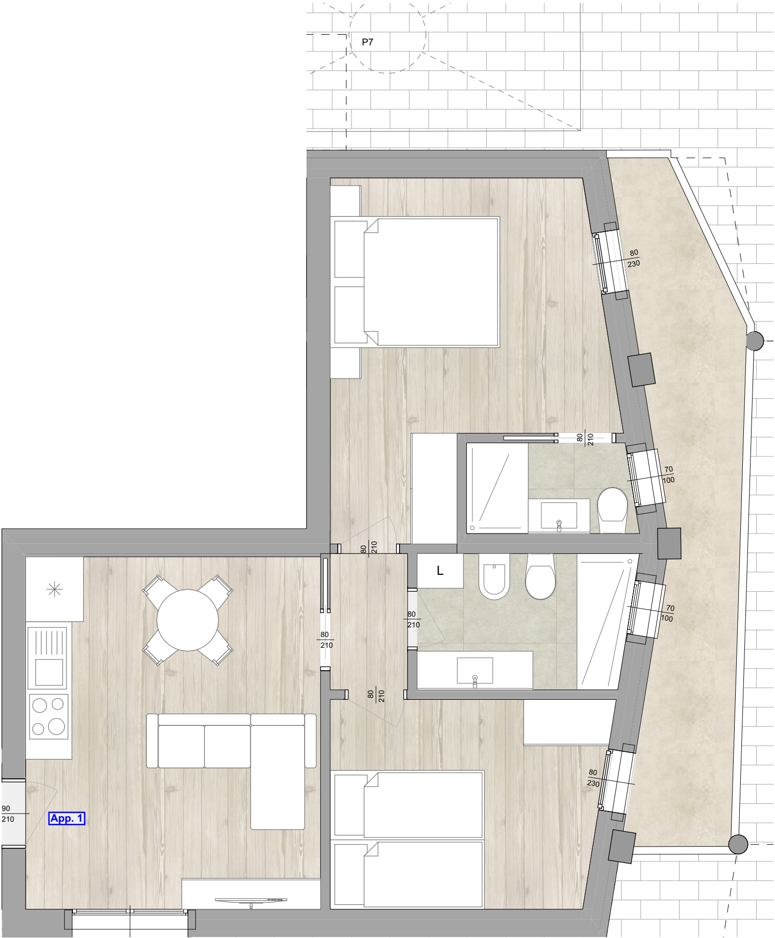
Appartamento 1
