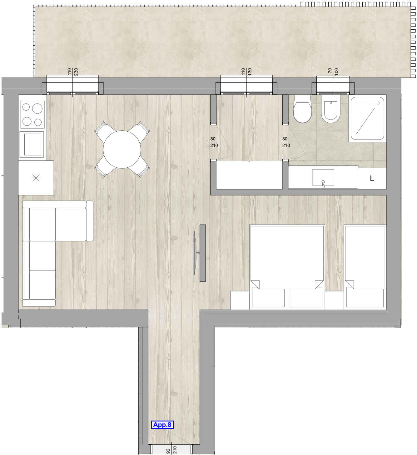
Appartamento 8 1:50
