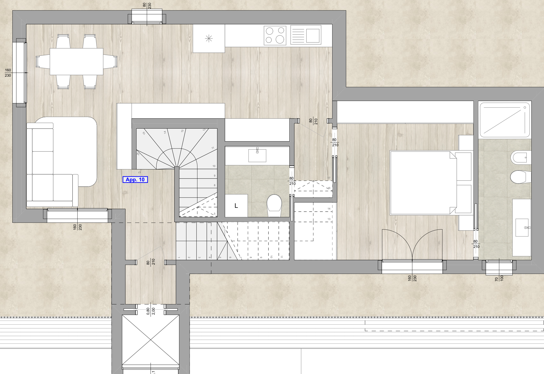
Appartamento 10
